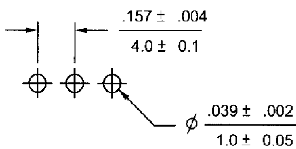
P.C.B. hole dimensions
