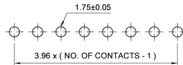
P.C.Board Layout
