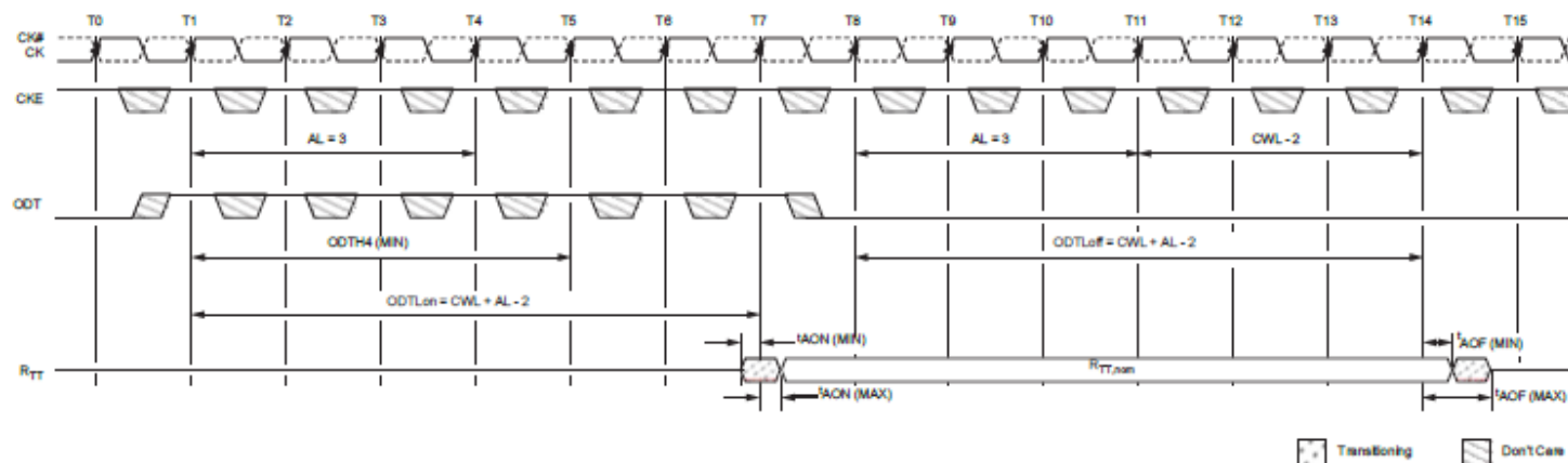
Figure 102 : Synchronous ODT
