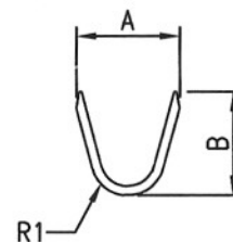
A-A SECTION
