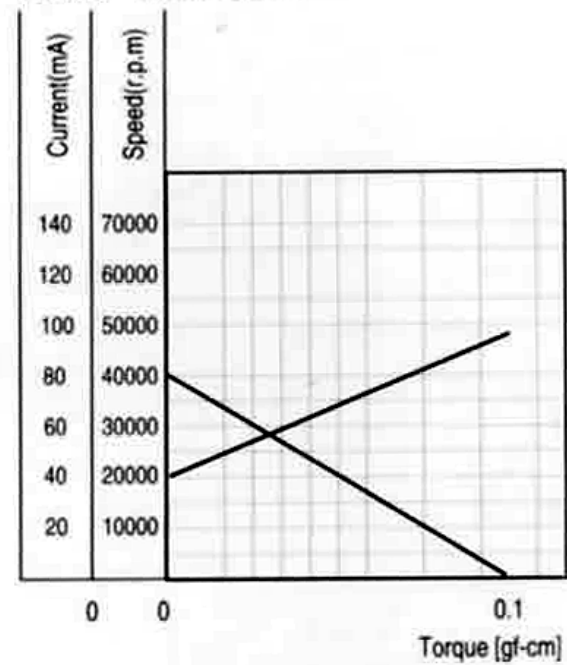
特性图 Characteristics
