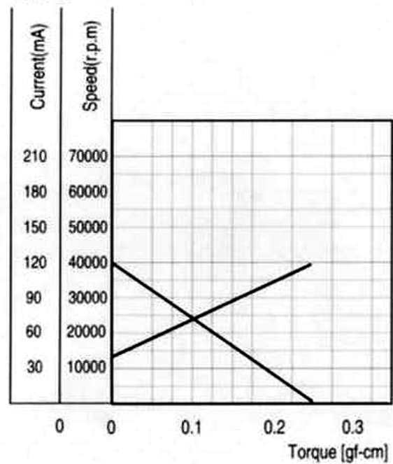
特性图 Characteristics
