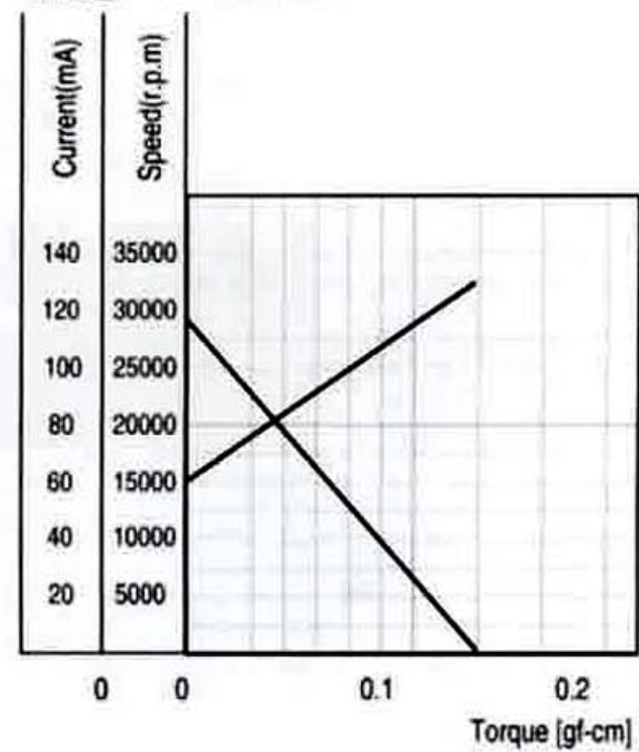
特性图 Characteristics
