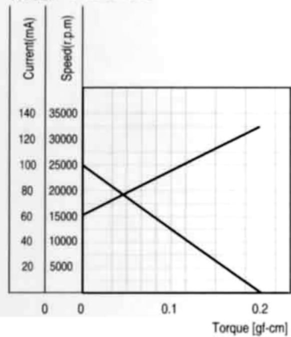
特性図 Characteristics
