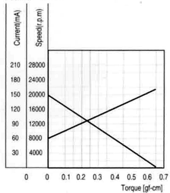
特性图 Characteristics
