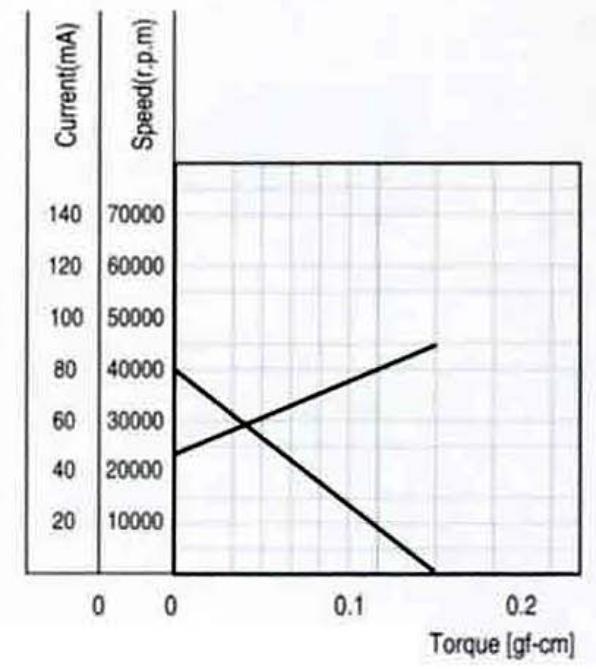
特性图 Characteristics
