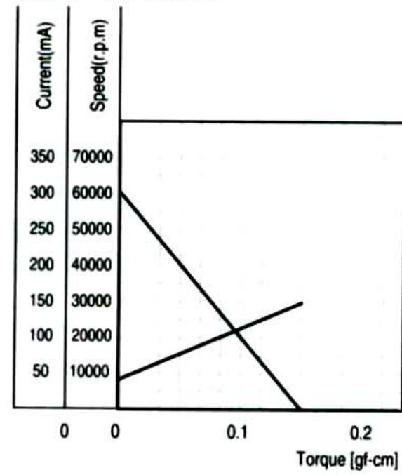
特性图 Characteristics
