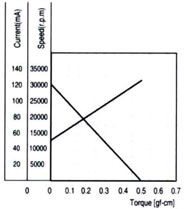
特性图 Characteristics
