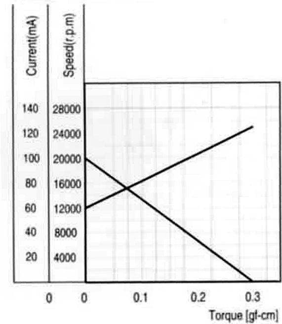
特性图 Characteristics
