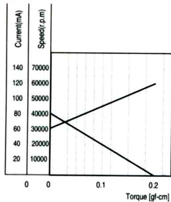
特性图 Characteristics
