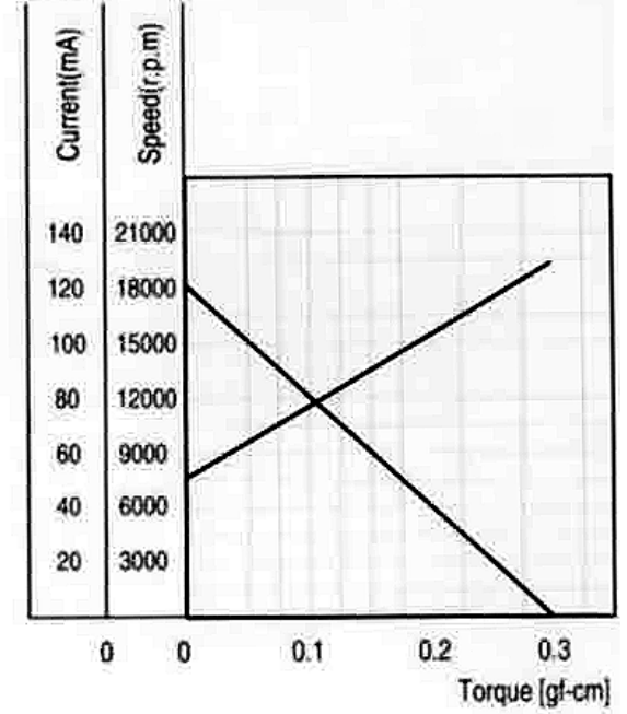
特性图 Characteristics
