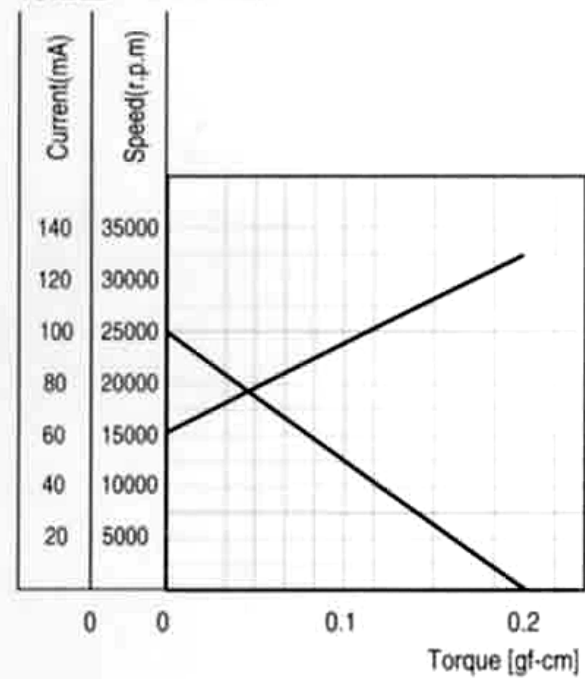
特性图 Characteristics
