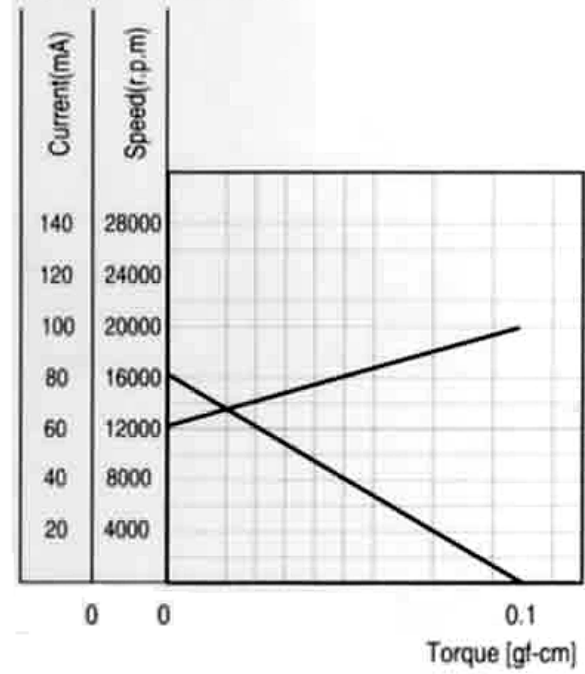
特性图 Characteristics
