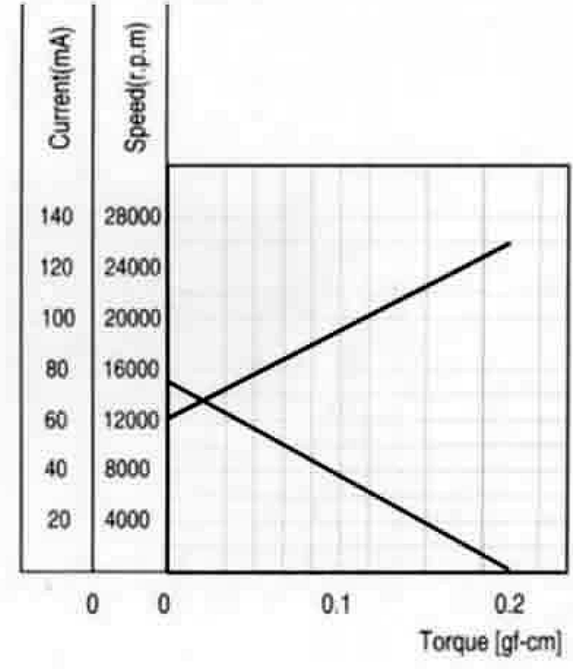
特性图 Characteristics
