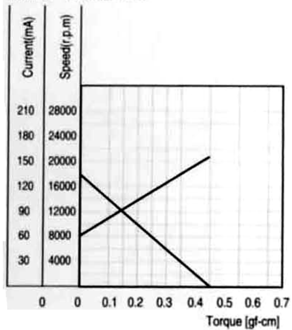
特性图 Characteristics
