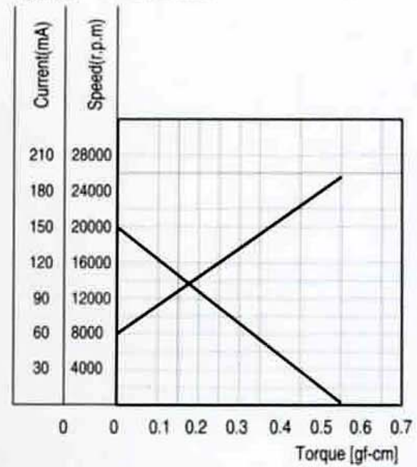
特性图 Characteristics
