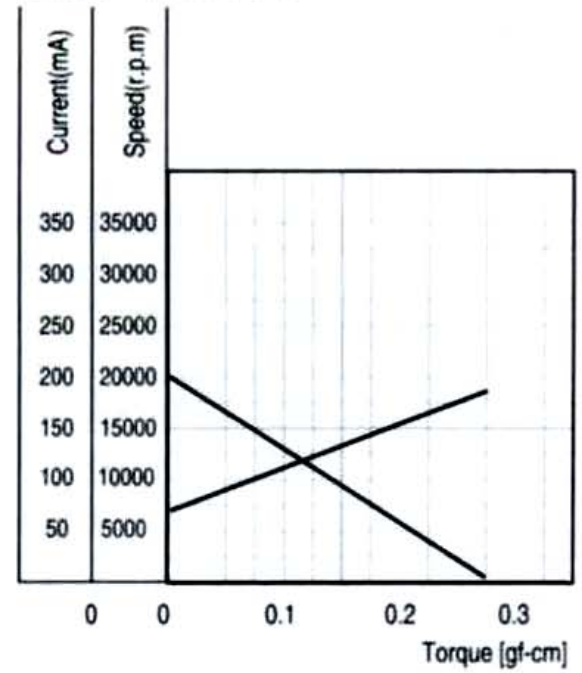
特性图 Characteristics
