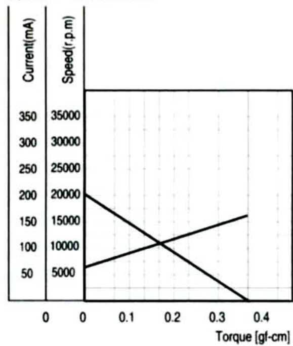
特性图 Characteristics
