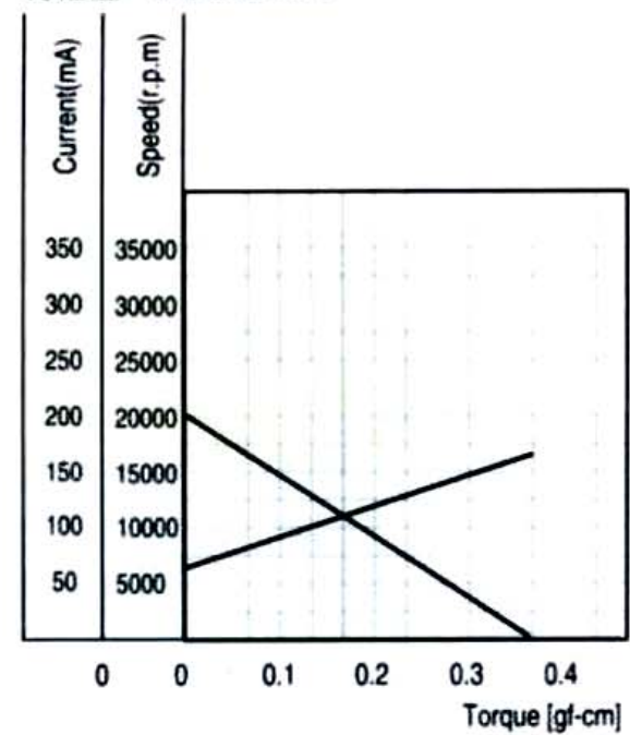
特性图 Characteristics
